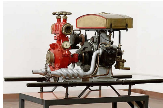
Tragkraftspritze B48, Fa. Rosenbauer
